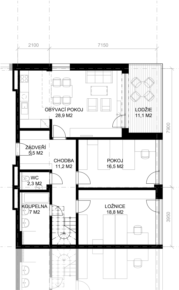
PŮDORYS 4.NP
