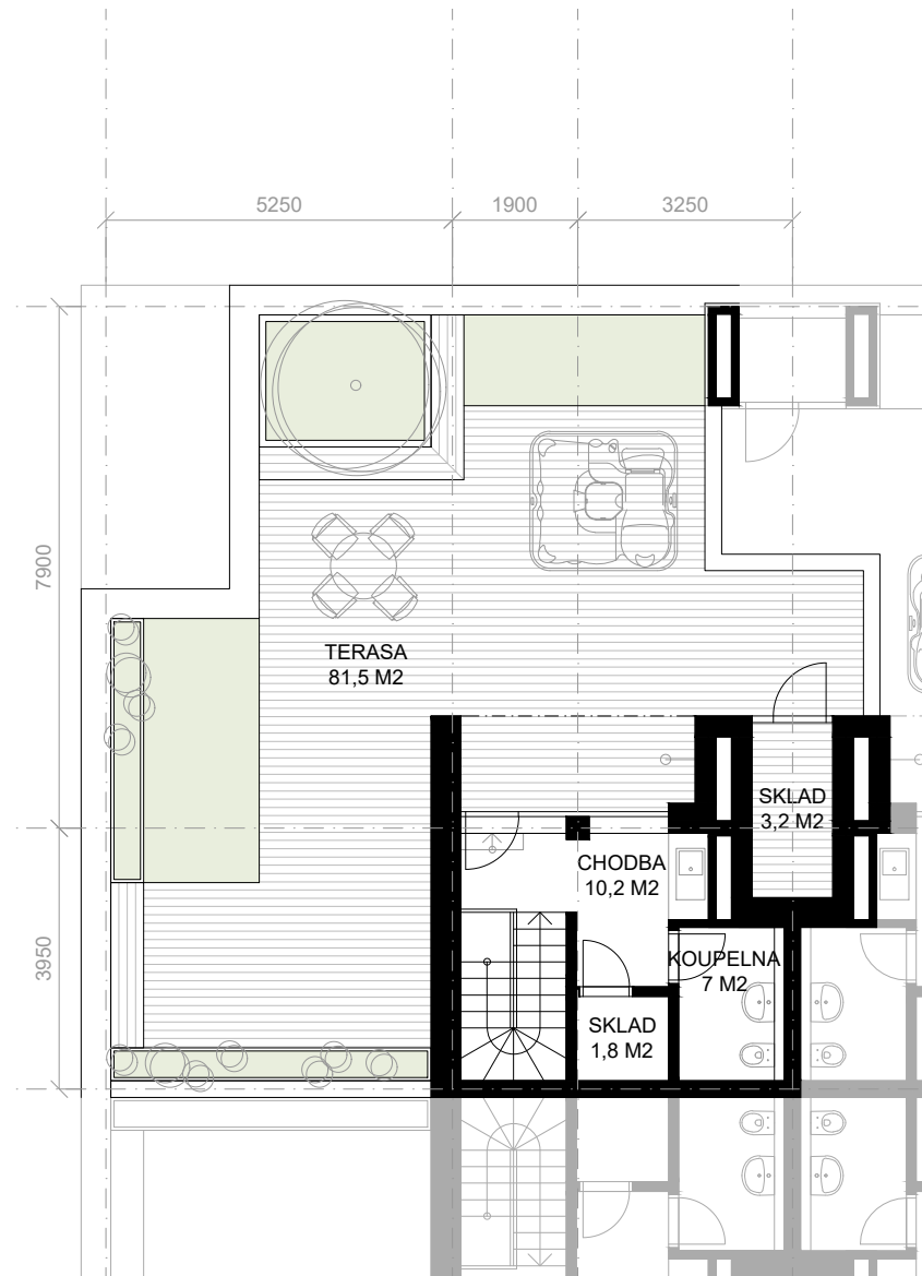
PŮDORYS 5.NP
