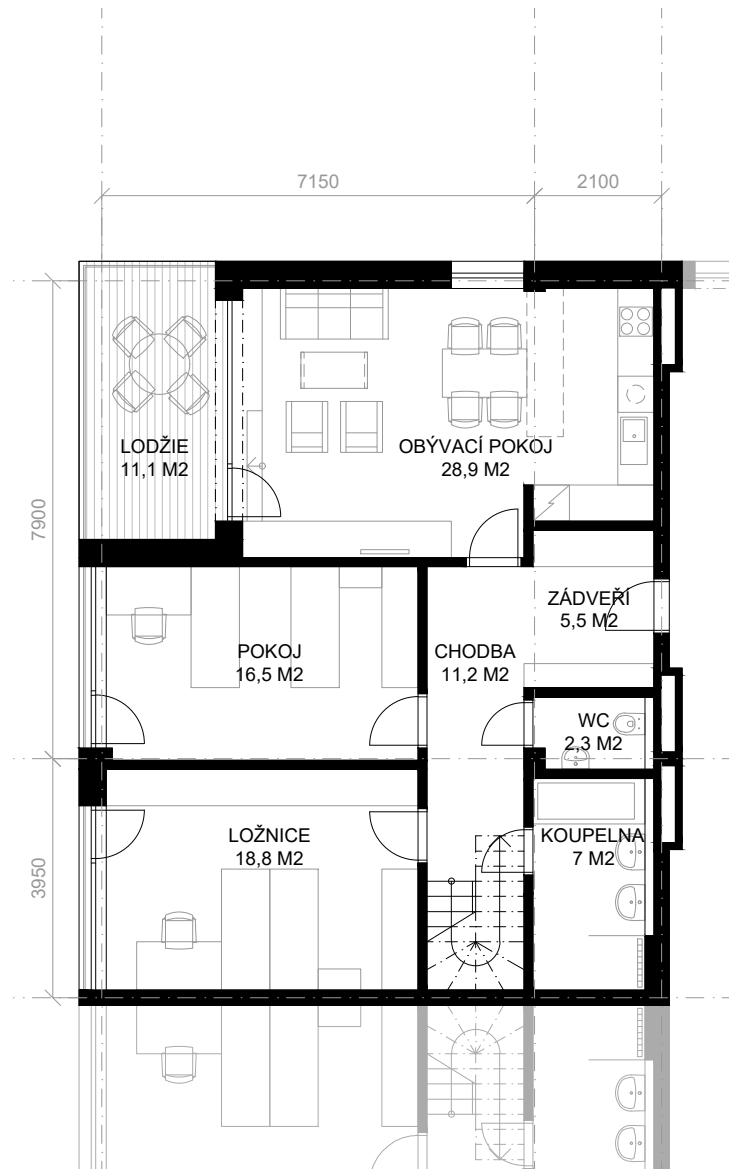
PŮDORYS 4.NP
