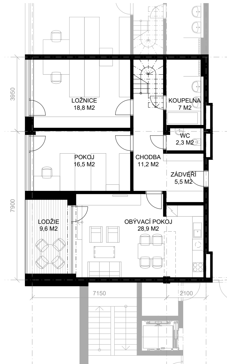
PŮDORYS 4.NP
